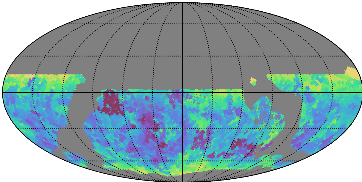
no_magell_roll_v3.4_10yrs WFD y band: Min seeingEff
