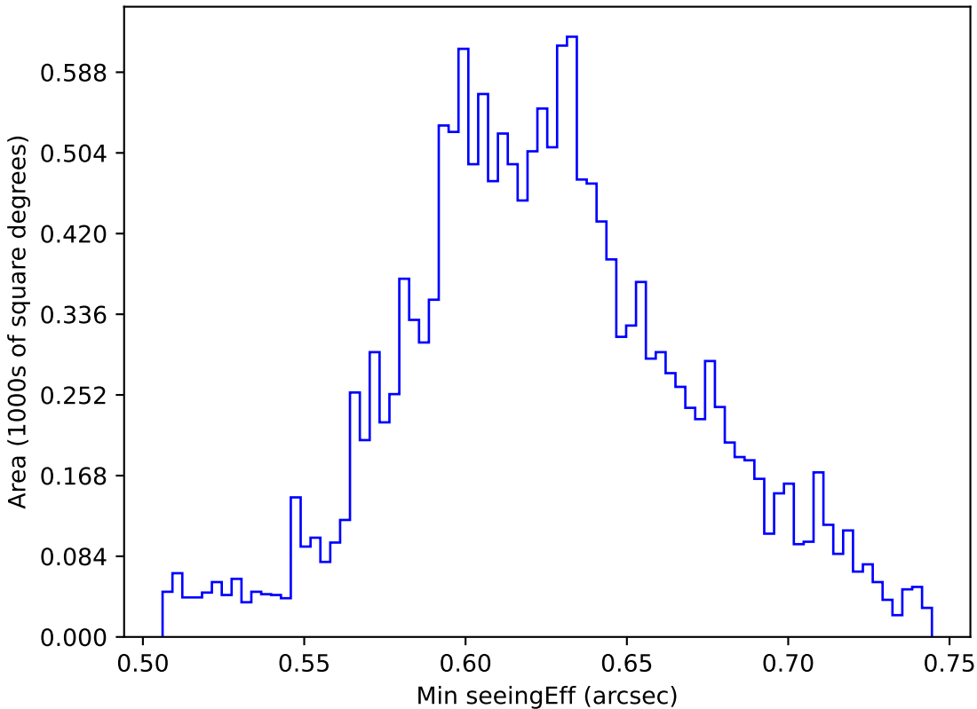
no_magell_roll_v3.4_10yrs WFD y band: Min seeingEff
