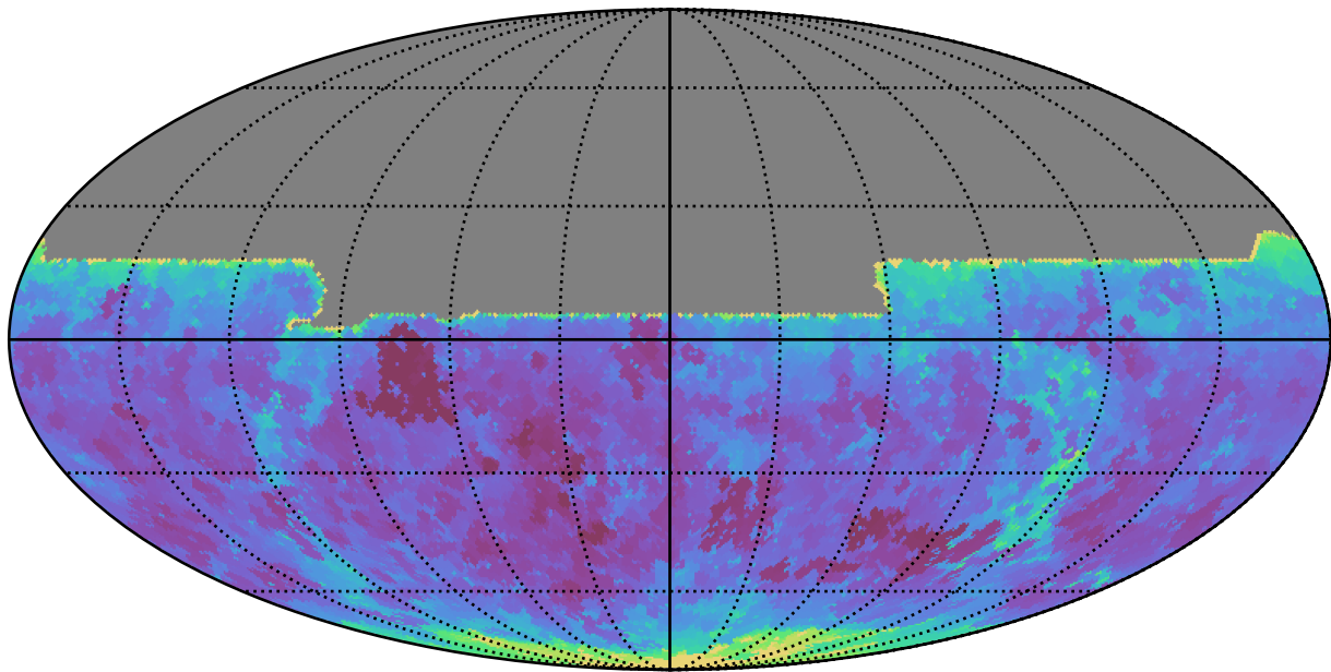
no_magell_roll_v3.4_10yrs All sky y band: Min seeingEff
