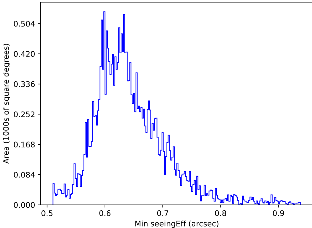
no_magell_roll_v3.4_10yrs All sky y band: Min seeingEff
