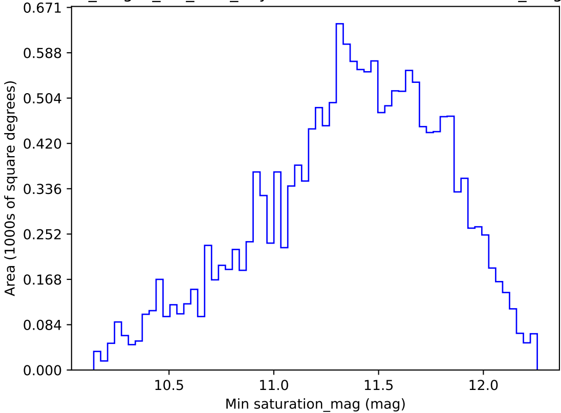
no_magell_roll_v3.4_10yrs WFD u band: Min saturation_mag
