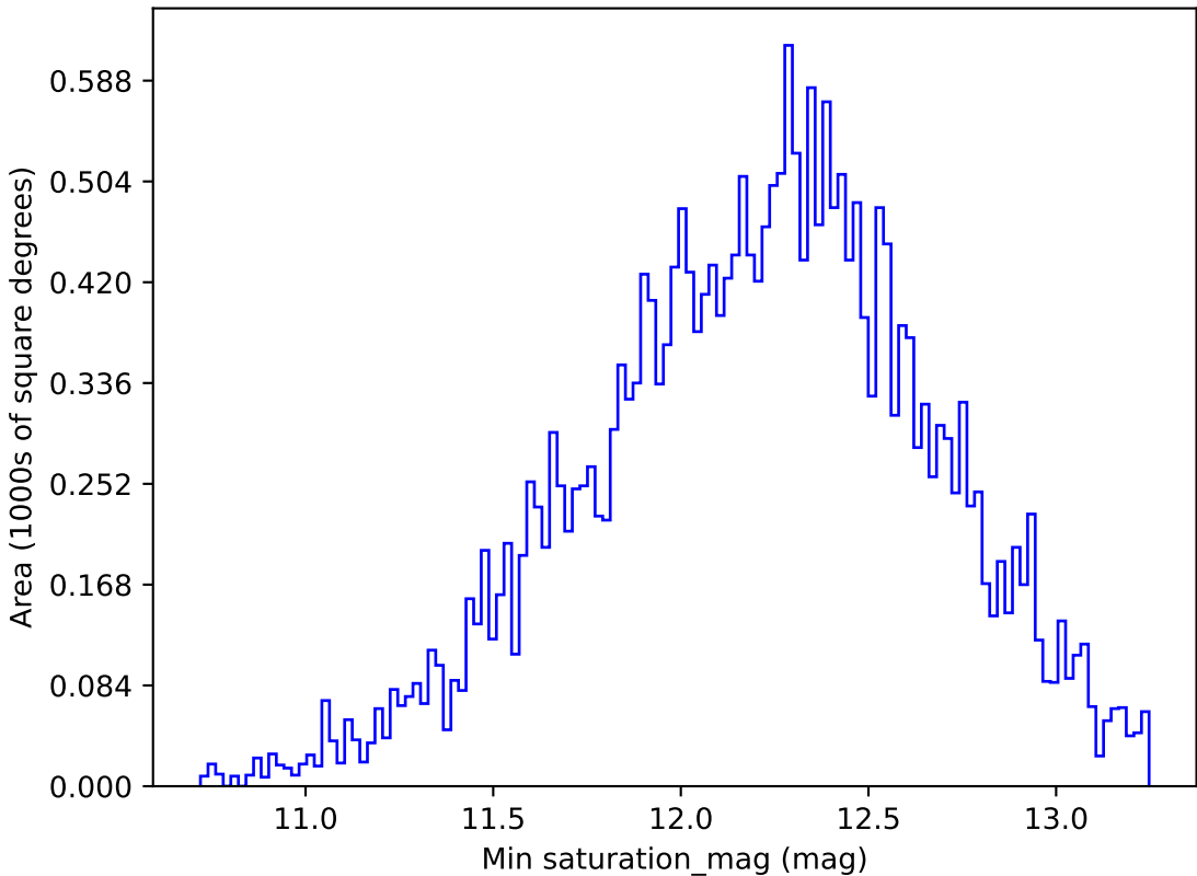
no_magell_roll_v3.4_10yrs All sky z band: Min saturation_mag
