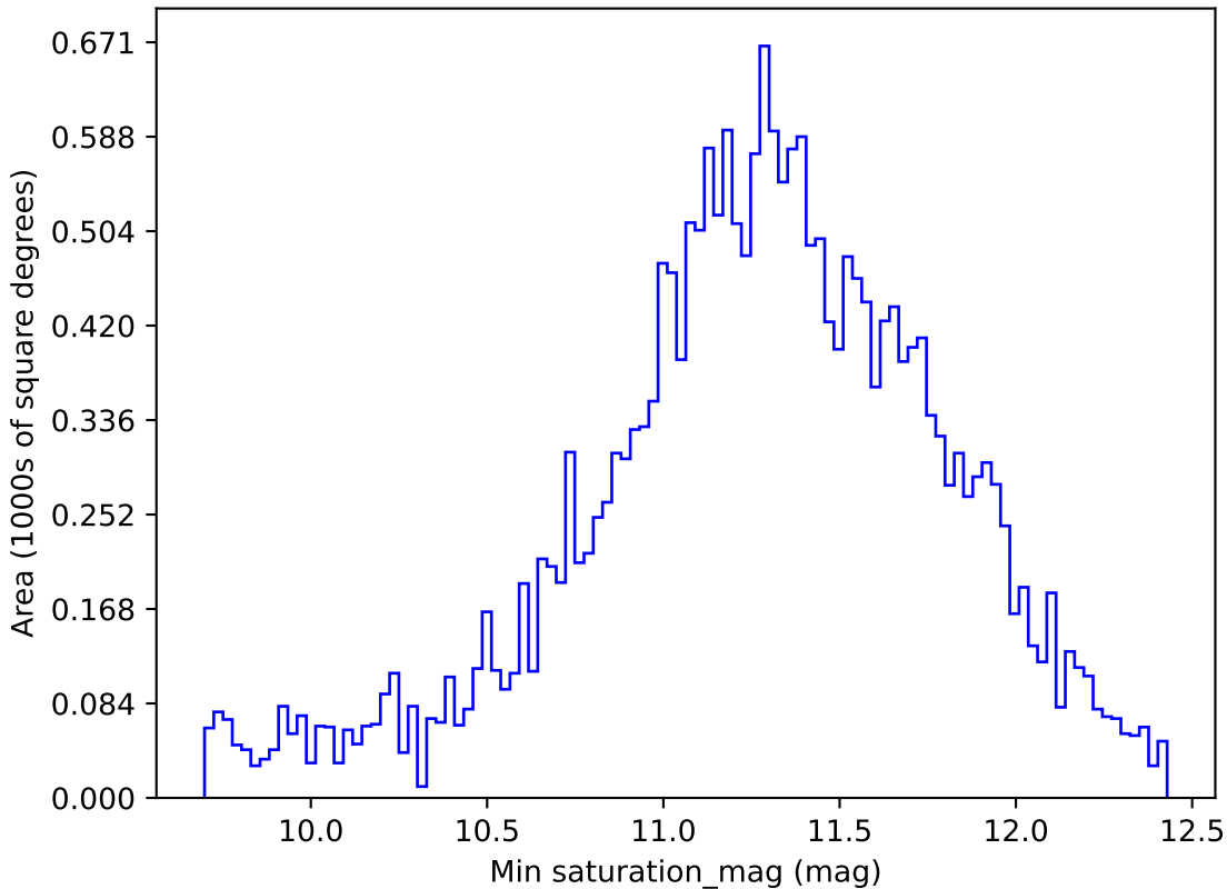
no_magell_roll_v3.4_10yrs All sky y band: Min saturation_mag
