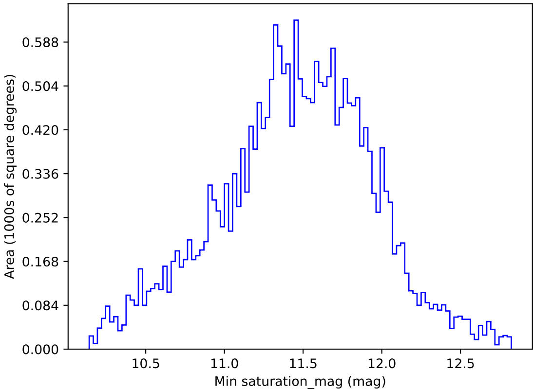
no_magell_roll_v3.4_10yrs All sky u band: Min saturation_mag
