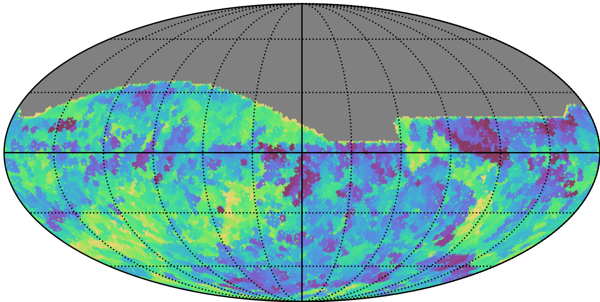
no_magell_roll_v3.4_10yrs All sky r band: Min saturation_mag
