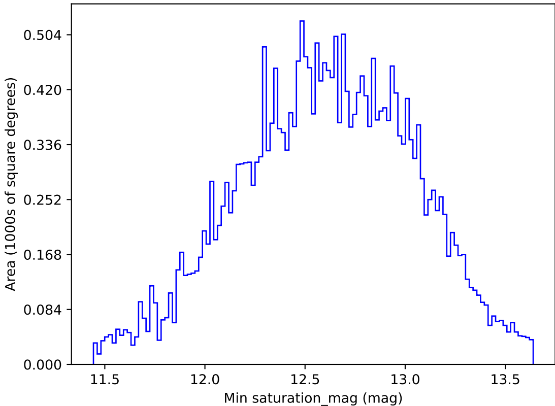
no_magell_roll_v3.4_10yrs All sky r band: Min saturation_mag
