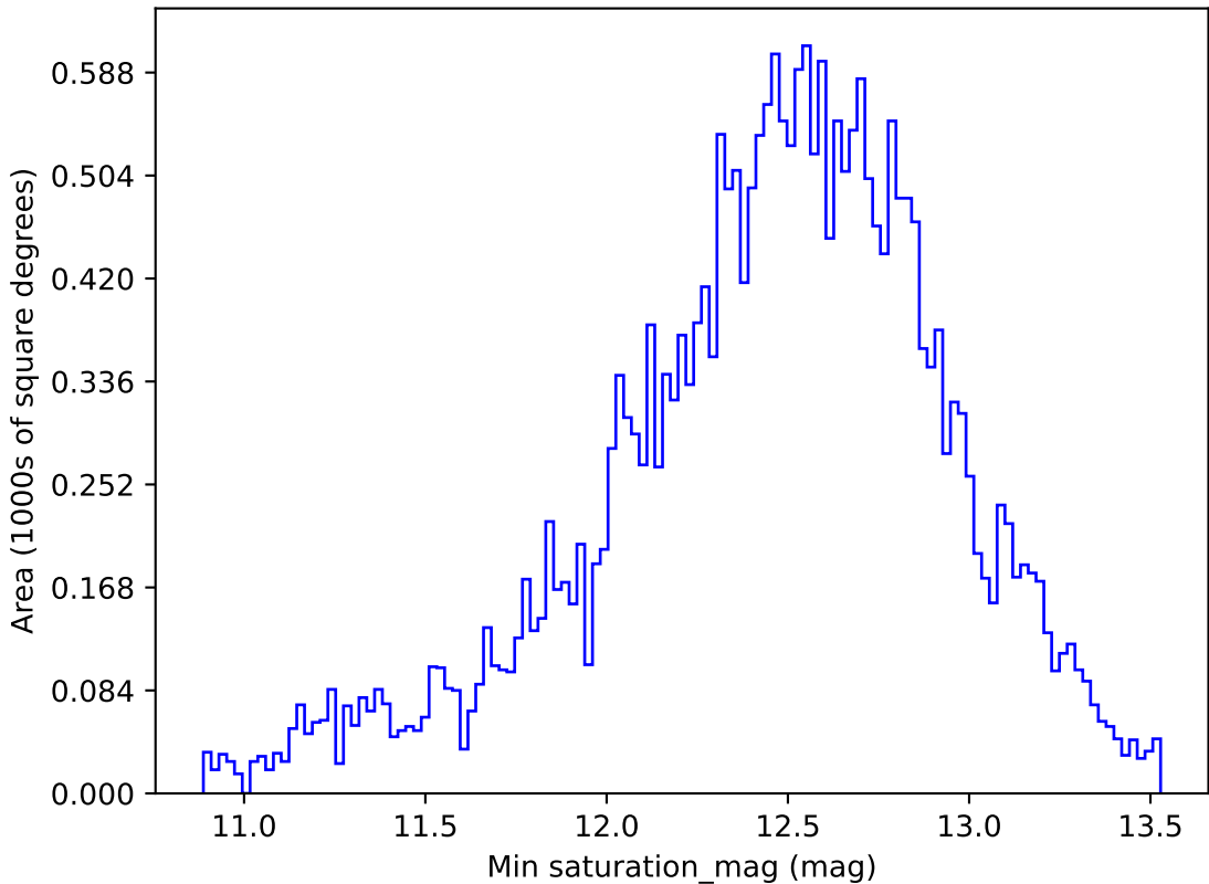
no_magell_roll_v3.4_10yrs All sky i band: Min saturation_mag
