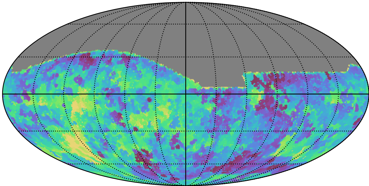
no_magell_roll_v3.4_10yrs All sky g band: Min saturation_mag
