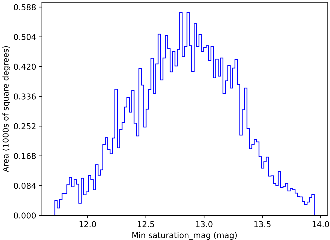
no_magell_roll_v3.4_10yrs All sky g band: Min saturation_mag
