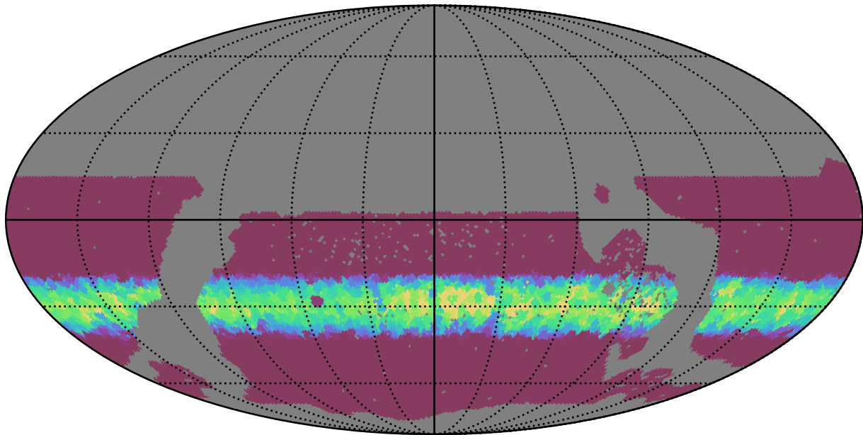
no_magell_roll_v3.4_10yrs WFD z band: Min normairmass
