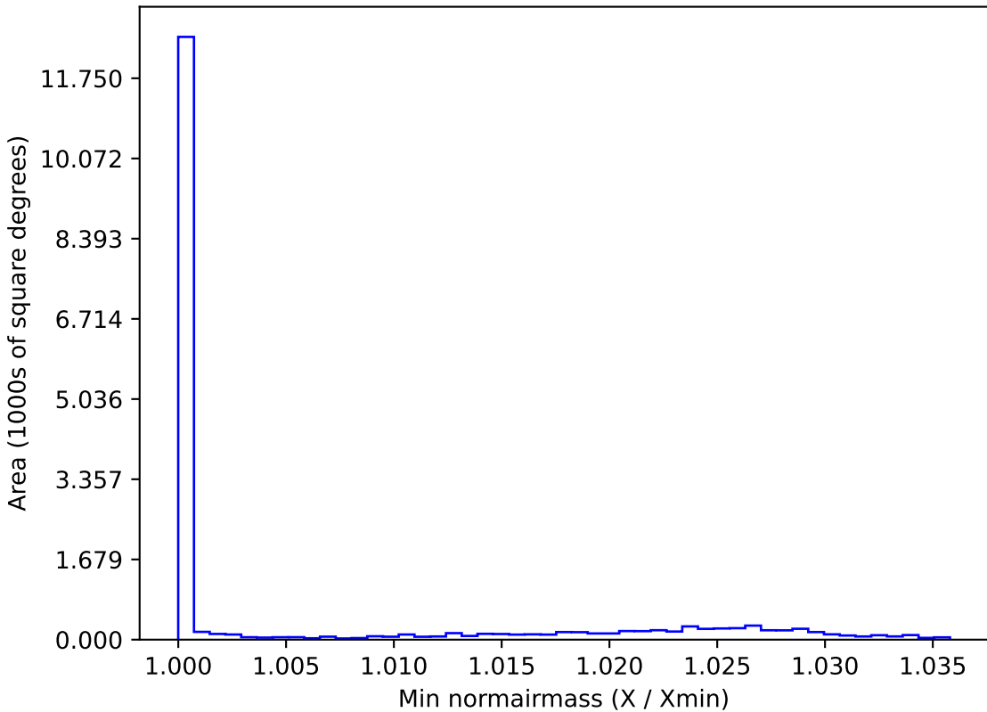
no_magell_roll_v3.4_10yrs WFD z band: Min normairmass
