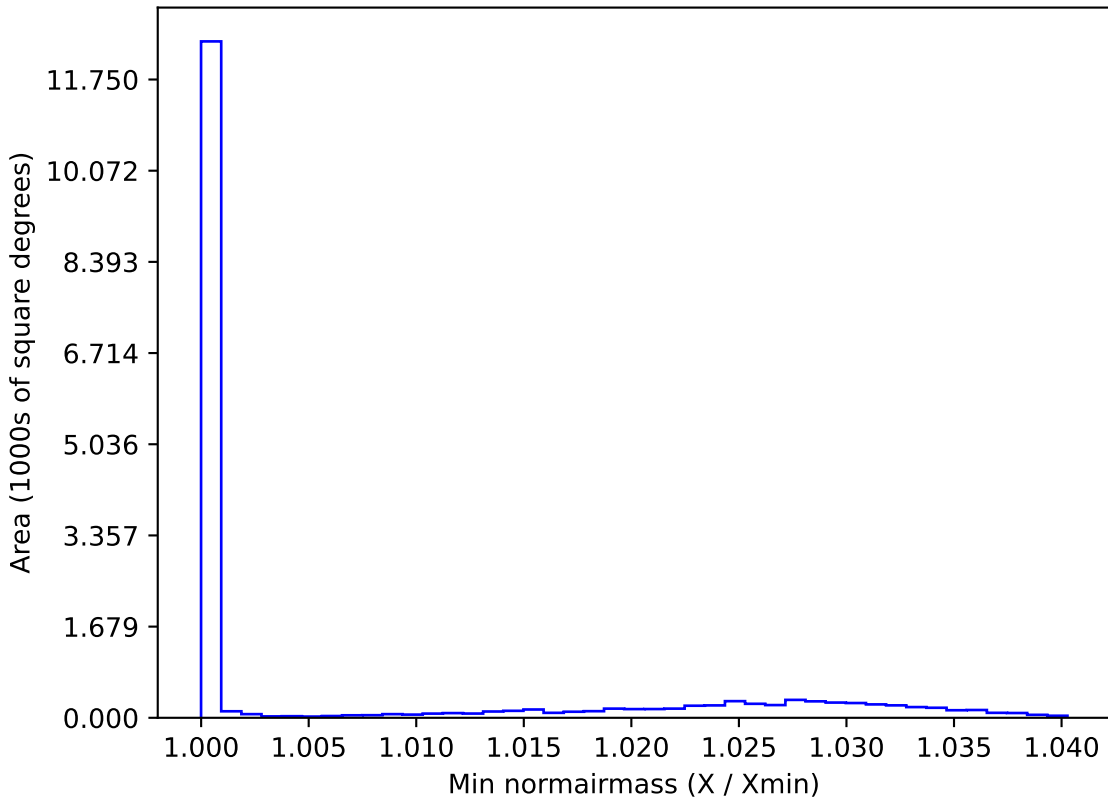
no_magell_roll_v3.4_10yrs WFD y band: Min normairmass
