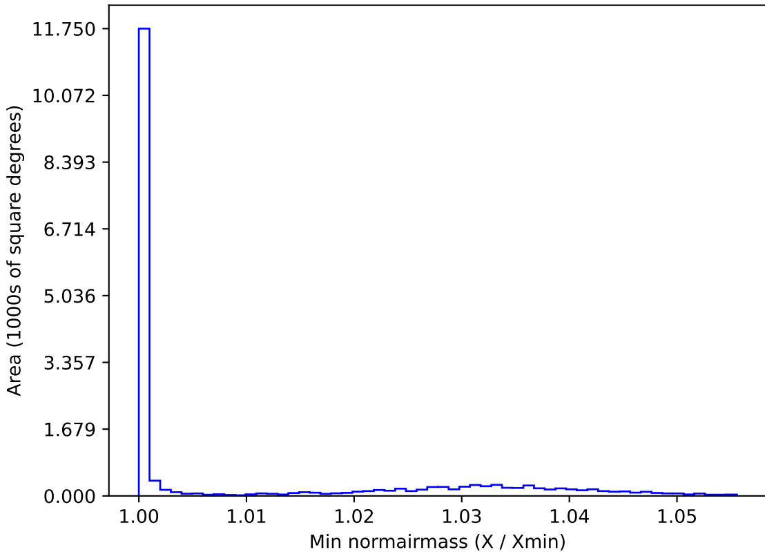
no_magell_roll_v3.4_10yrs WFD u band: Min normairmass
