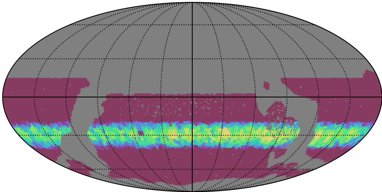
no_magell_roll_v3.4_10yrs WFD r band: Min normairmass
