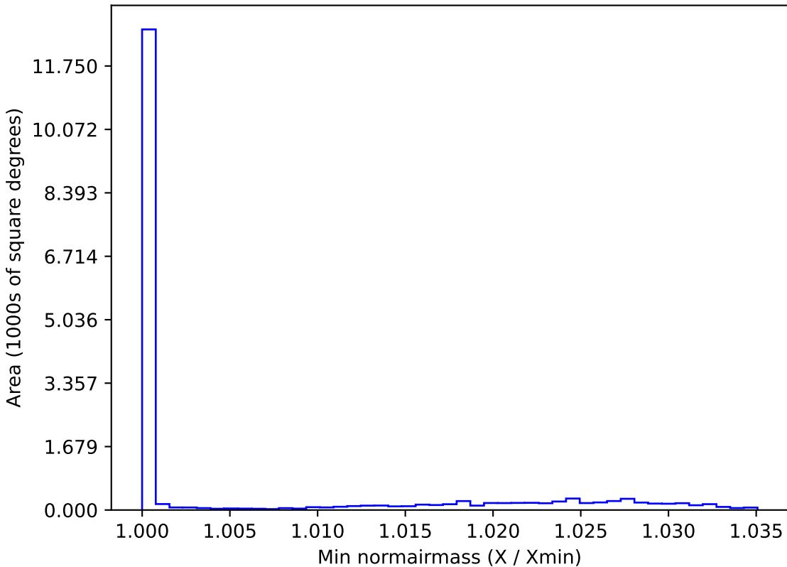
no_magell_roll_v3.4_10yrs WFD i band: Min normairmass
