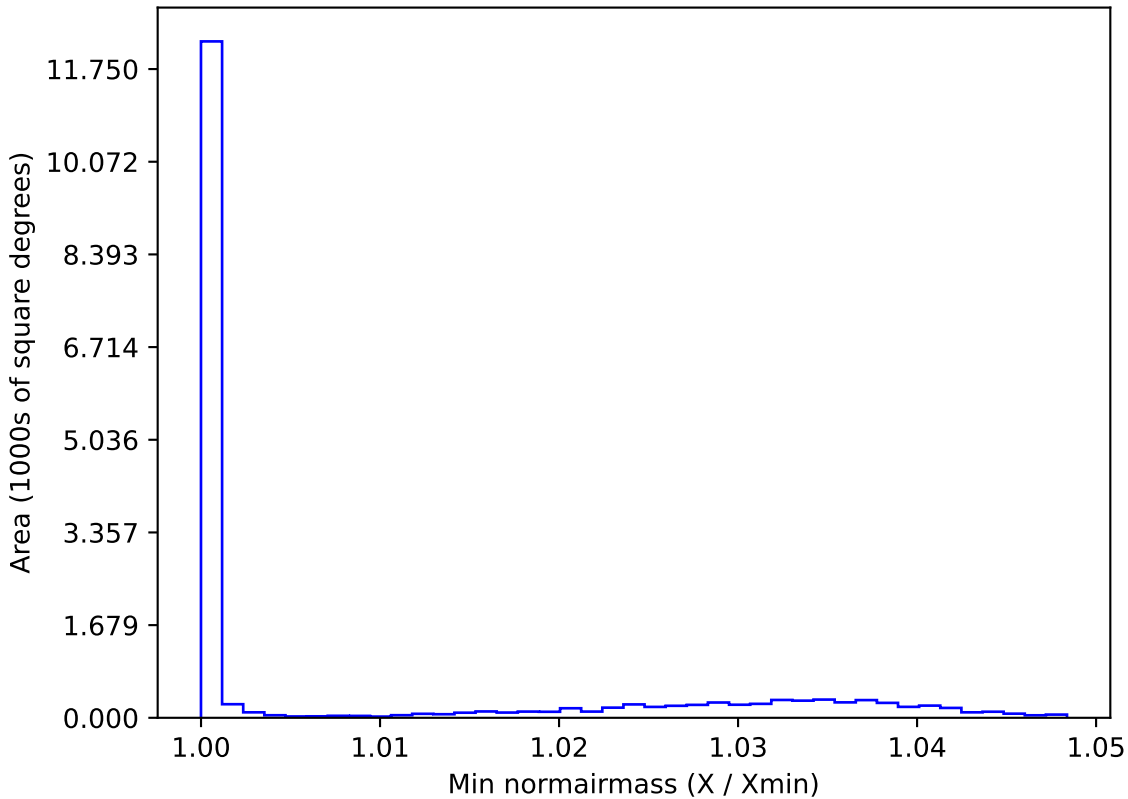
no_magell_roll_v3.4_10yrs WFD g band: Min normairmass
