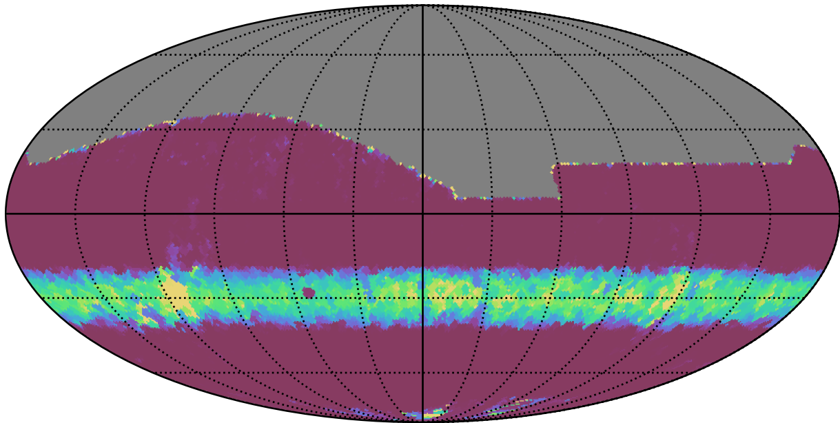
no_magell_roll_v3.4_10yrs All sky z band: Min normairmass
