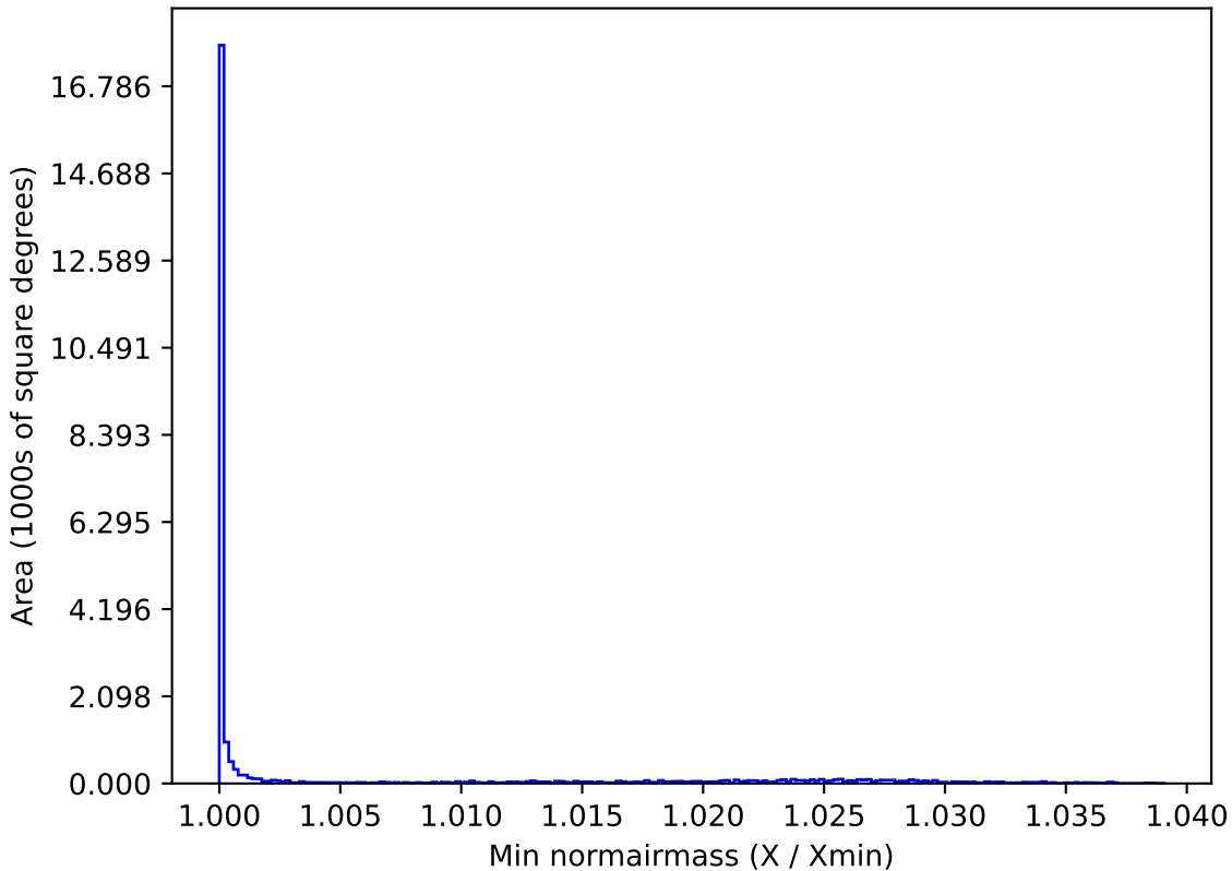
no_magell_roll_v3.4_10yrs All sky z band: Min normairmass
