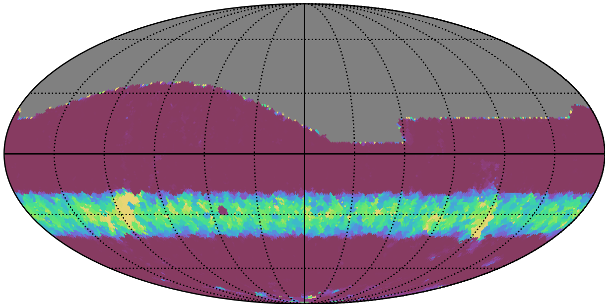
no_magell_roll_v3.4_10yrs All sky g band: Min normairmass
