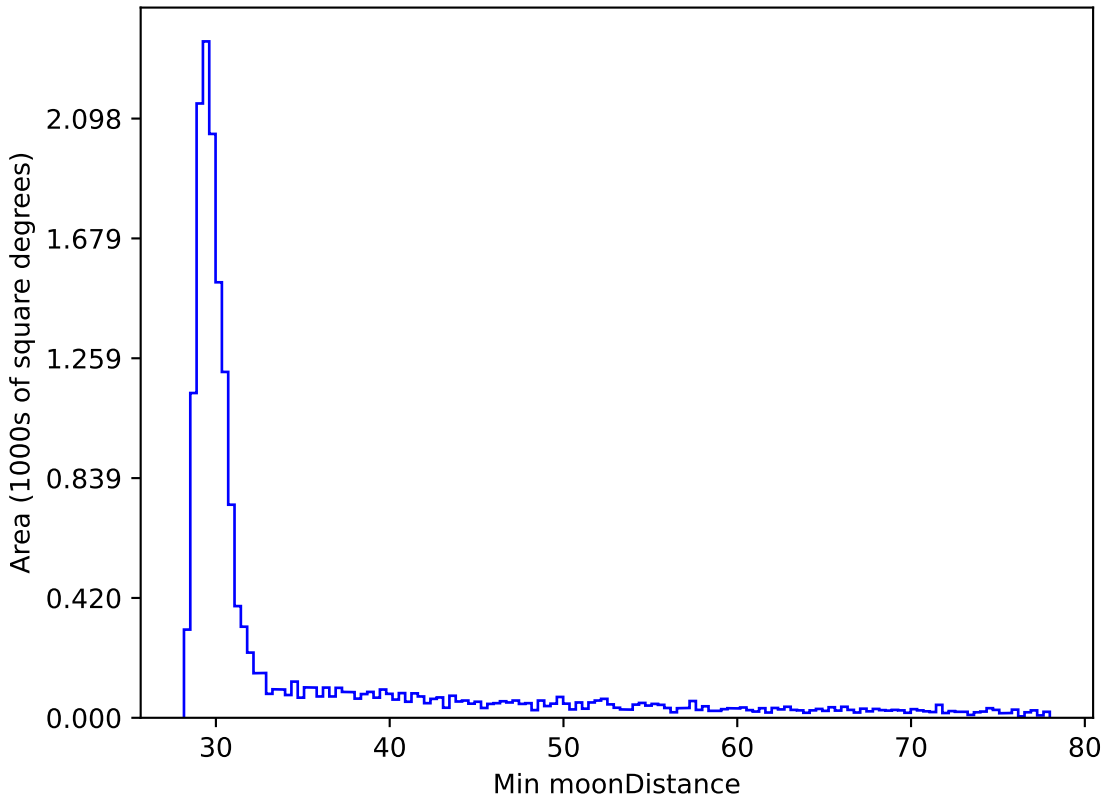
no_magell_roll_v3.4_10yrs WFD z band: Min moonDistance
