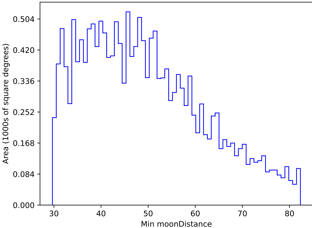
no_magell_roll_v3.4_10yrs WFD u band: Min moonDistance
