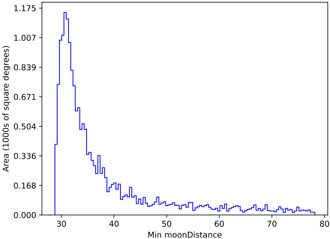
no_magell_roll_v3.4_10yrs WFD r band: Min moonDistance
