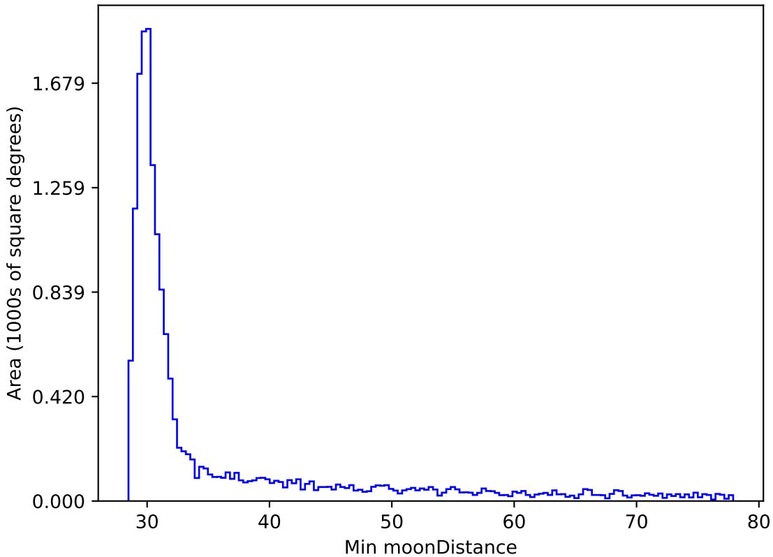
no_magell_roll_v3.4_10yrs WFD i band: Min moonDistance
