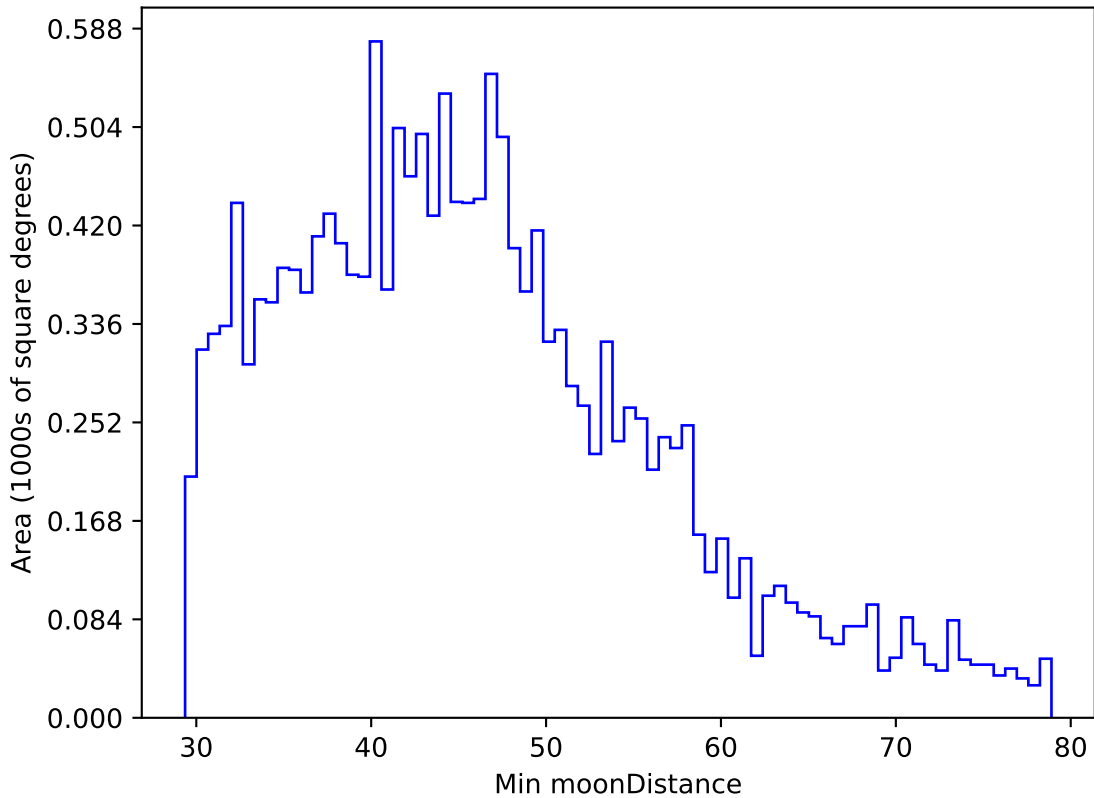
no_magell_roll_v3.4_10yrs WFD g band: Min moonDistance
