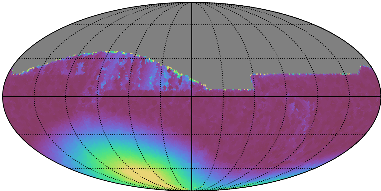
no_magell_roll_v3.4_10yrs All sky z band: Min moonDistance
