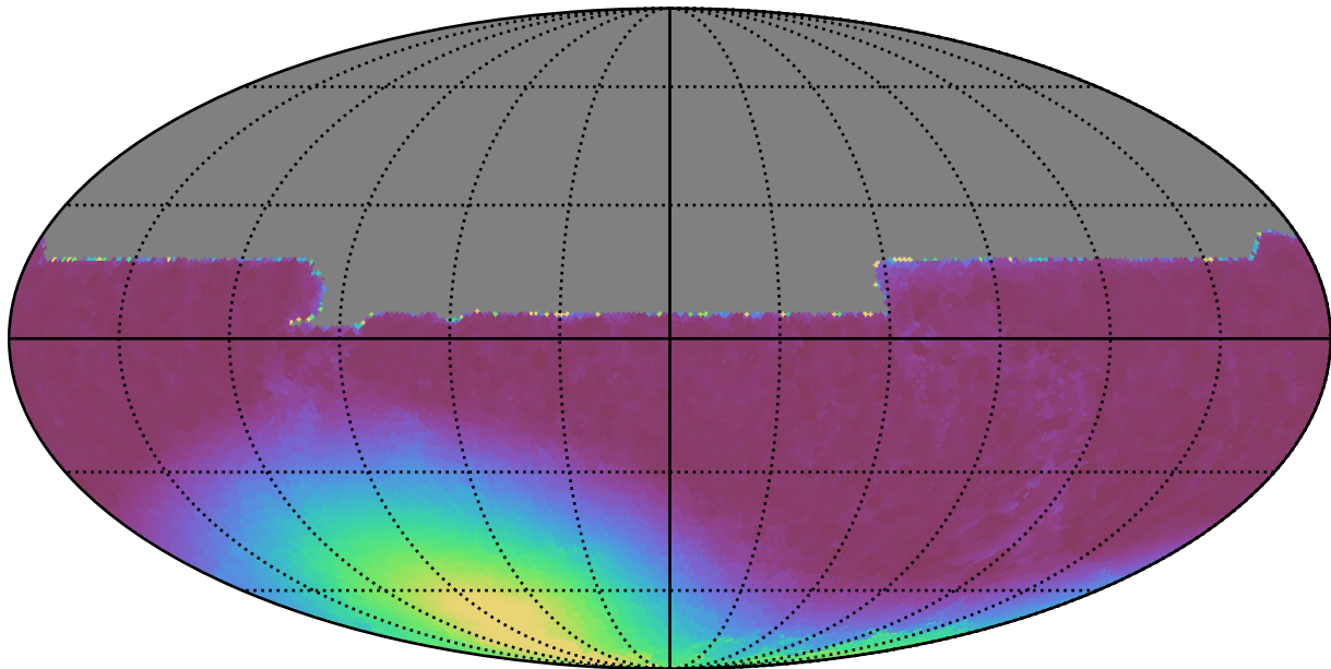
no_magell_roll_v3.4_10yrs All sky y band: Min moonDistance
