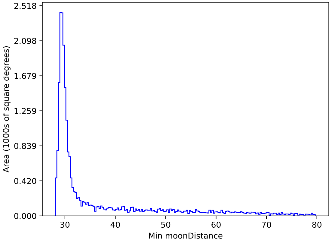
no_magell_roll_v3.4_10yrs All sky y band: Min moonDistance
