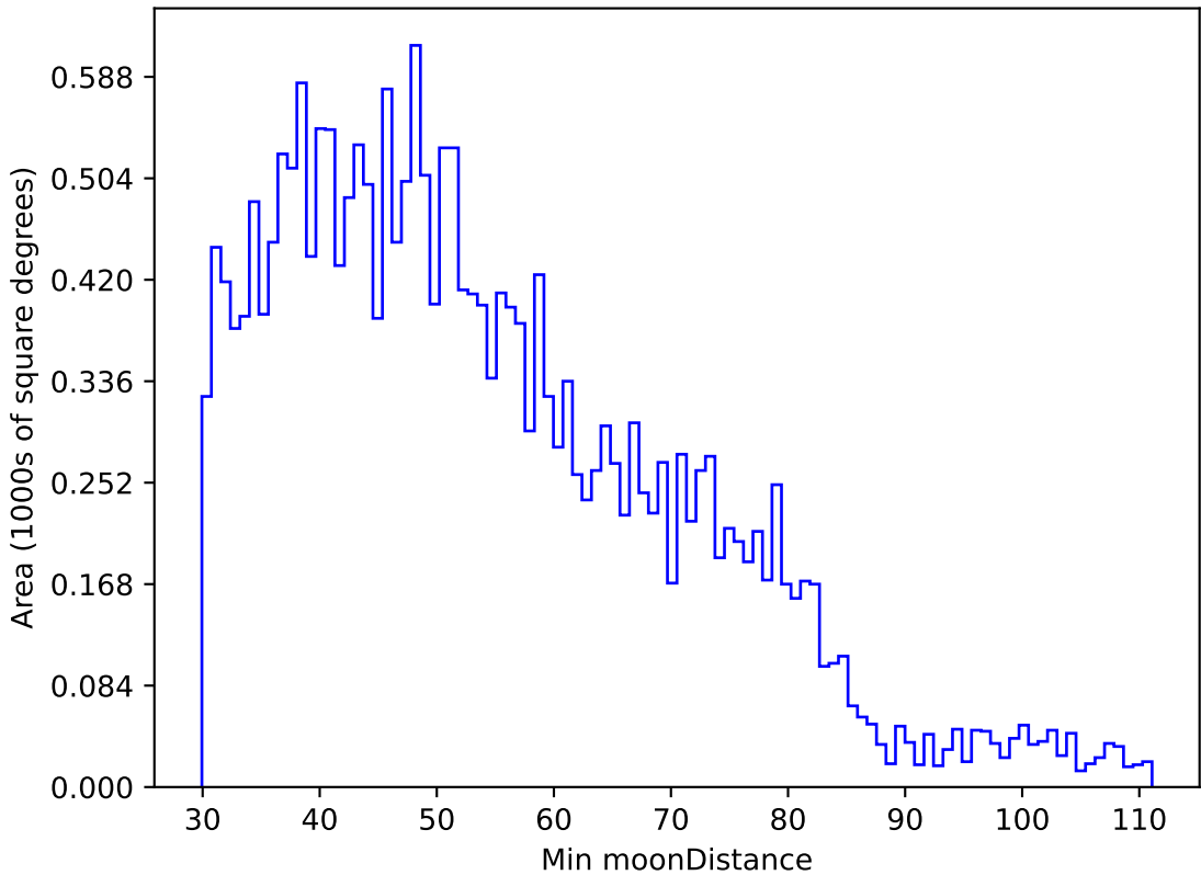
no_magell_roll_v3.4_10yrs All sky u band: Min moonDistance
