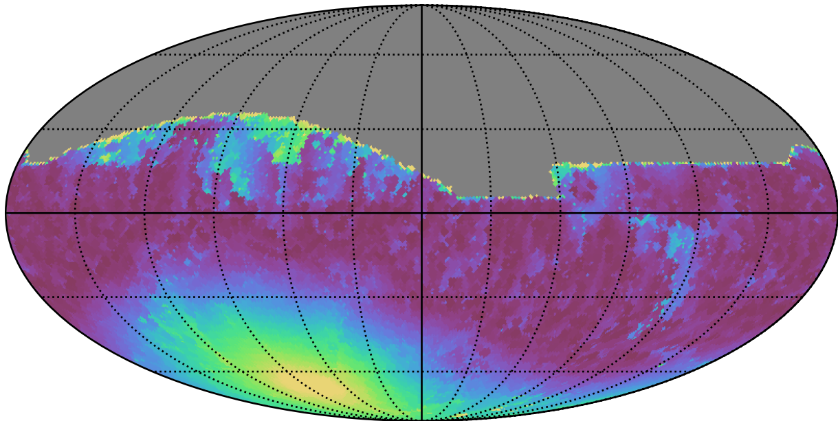
no_magell_roll_v3.4_10yrs All sky r band: Min moonDistance
