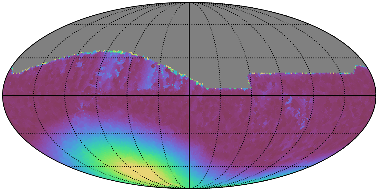
no_magell_roll_v3.4_10yrs All sky i band: Min moonDistance
