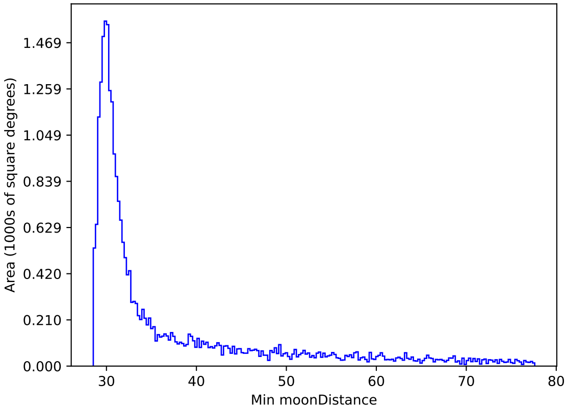
no_magell_roll_v3.4_10yrs All sky i band: Min moonDistance
