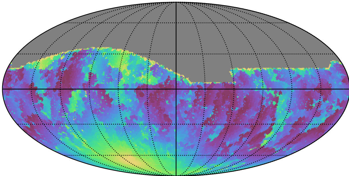
no_magell_roll_v3.4_10yrs All sky g band: Min moonDistance
