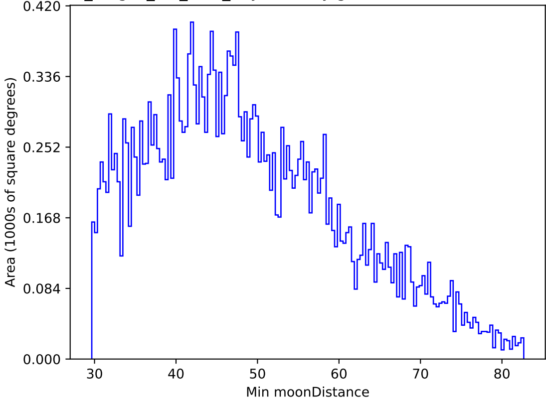
no_magell_roll_v3.4_10yrs All sky g band: Min moonDistance
