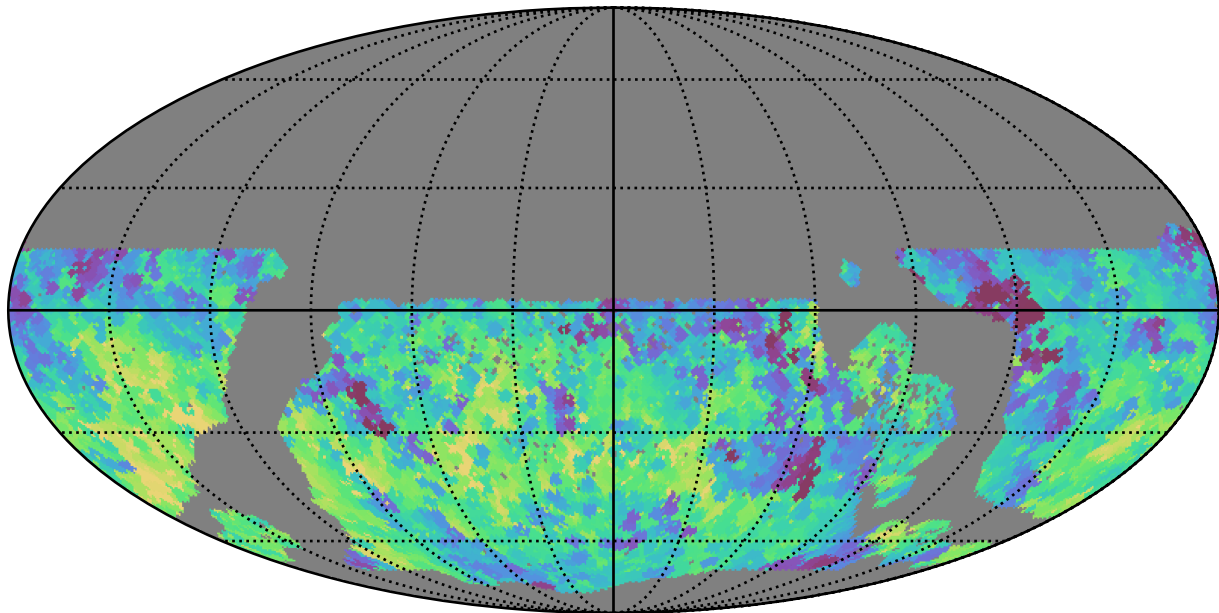
no_magell_roll_v3.4_10yrs WFD y band: Min fiveSigmaDepth
