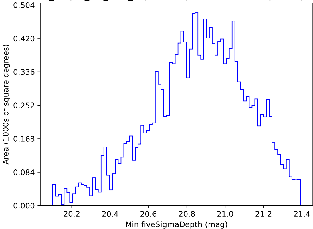
no_magell_roll_v3.4_10yrs WFD y band: Min fiveSigmaDepth
