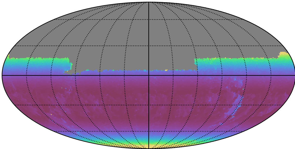
no_magell_roll_v3.4_10yrs Yr 1 y band: Min airmass
