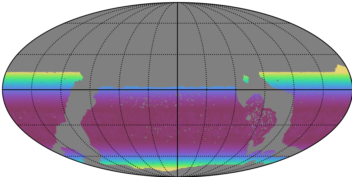
no_magell_roll_v3.4_10yrs WFD y band: Min airmass
