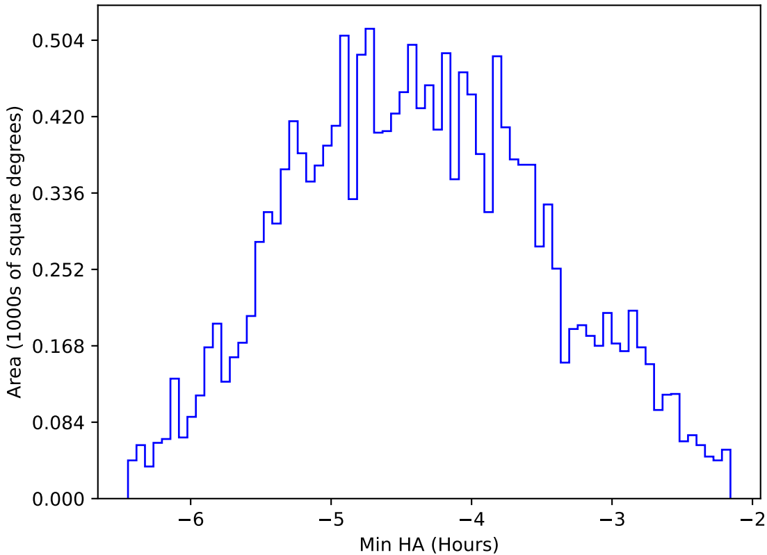
no_magell_roll_v3.4_10yrs WFD z band: Min HA
