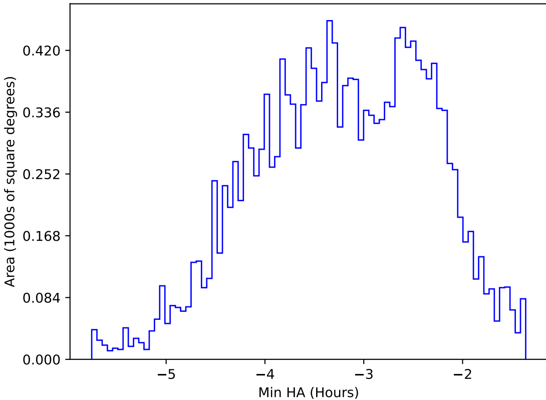
no_magell_roll_v3.4_10yrs WFD u band: Min HA
