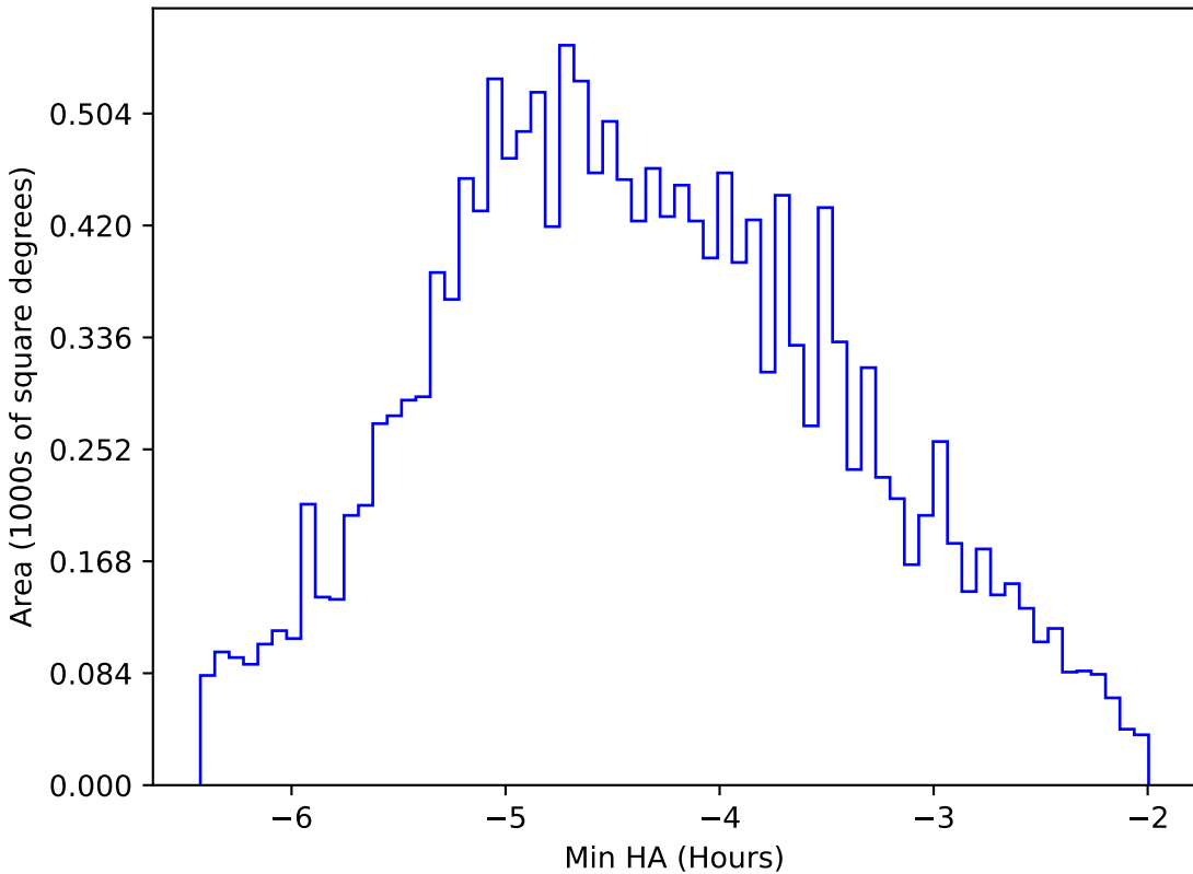
no_magell_roll_v3.4_10yrs WFD i band: Min HA
