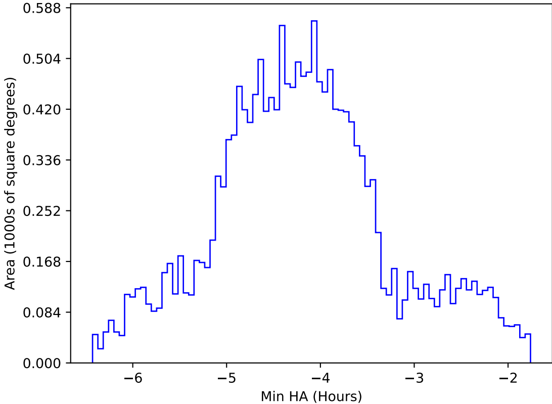
no_magell_roll_v3.4_10yrs WFD g band: Min HA
