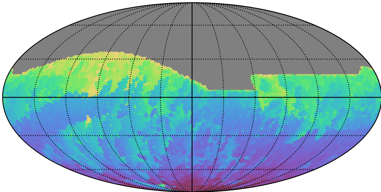
no_magell_roll_v3.4_10yrs All sky z band: Min HA
