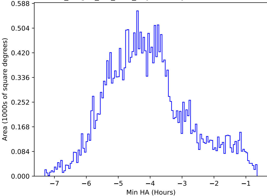
no_magell_roll_v3.4_10yrs All sky z band: Min HA
