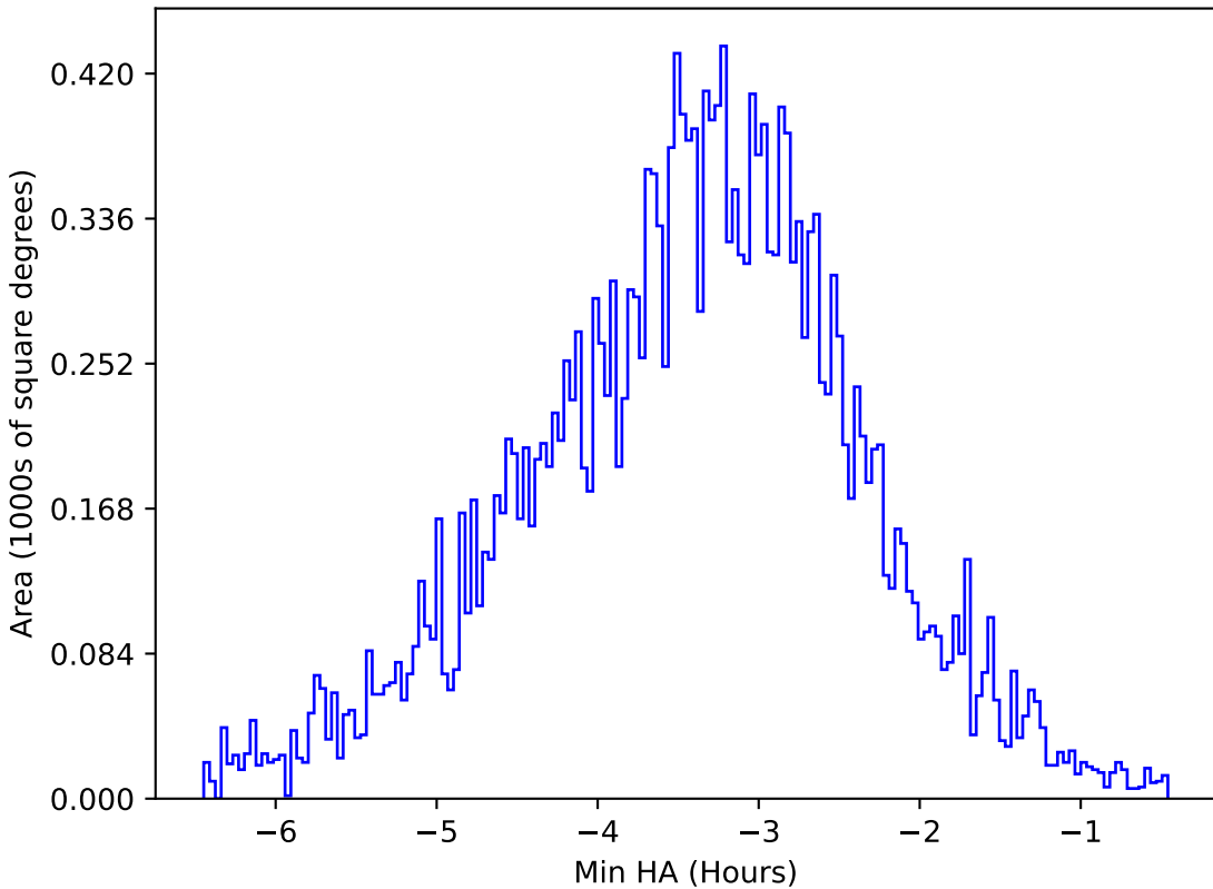
no_magell_roll_v3.4_10yrs All sky y band: Min HA
