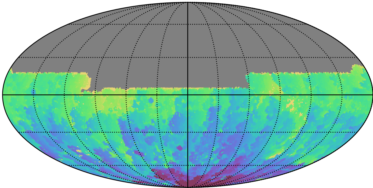
no_magell_roll_v3.4_10yrs All sky u band: Min HA
