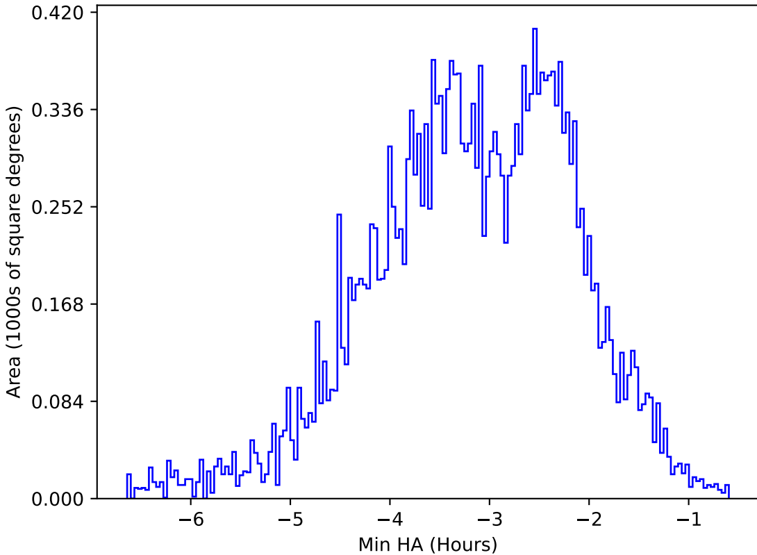
no_magell_roll_v3.4_10yrs All sky u band: Min HA
